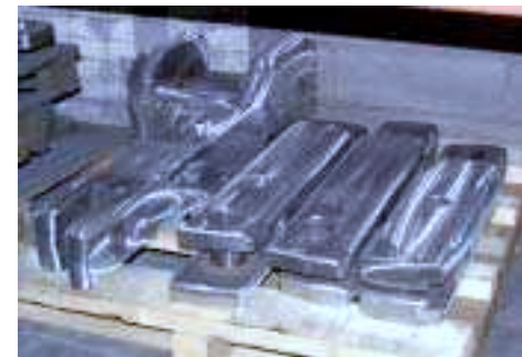
MAILLONS DE CHAINE DE MANNEQUIN DE COULEE CONTINUE ET REPARATION
