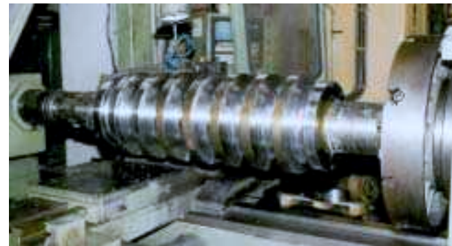
ROULEAU DE TABLE EN COURS DE TOURNAGE
