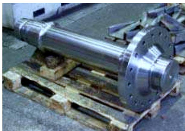
DIFFERENTS TYPES D'ALLONGES POUR LAMINOIRS
