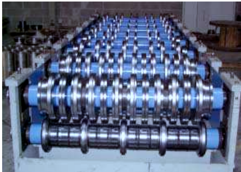
Galets Ø150 à 250 mm réalisés en Z155CDV12 traités 58/60HRC avec entretoises
