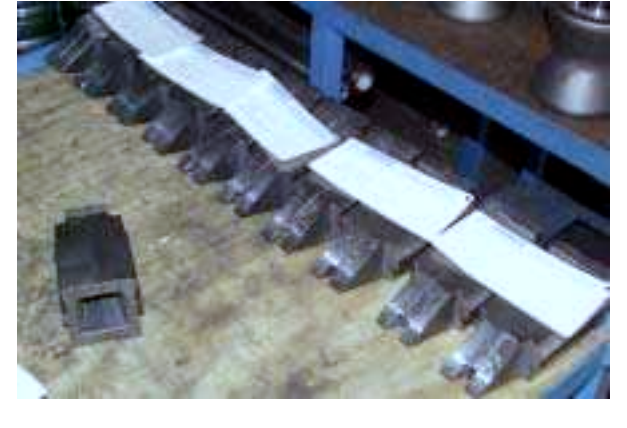
Halbe Führungen und Düsen für die Drahtindustrie
